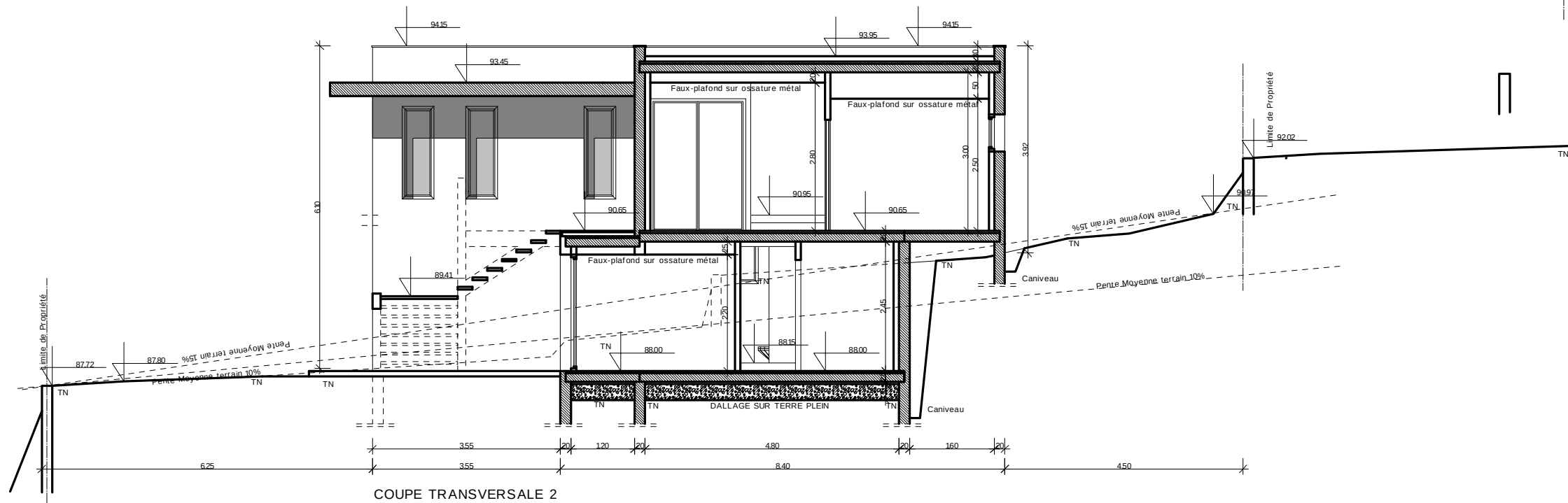
COUPE TRANSVERSALE 2
